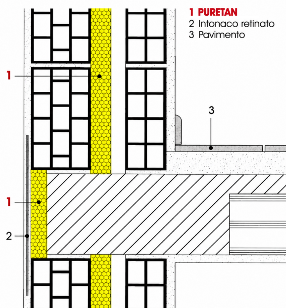
Isolamento termico dall'interno controfodera
