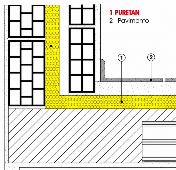
Isolamento sotto pavimentazione solai intermedi
